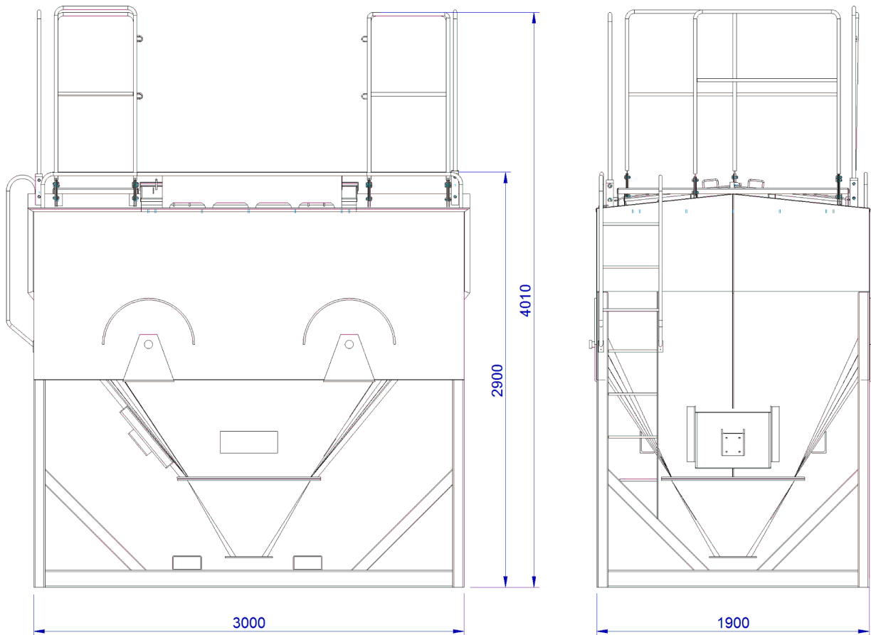
HUVUDMÅTT STORBEHÅLLARE SP10
