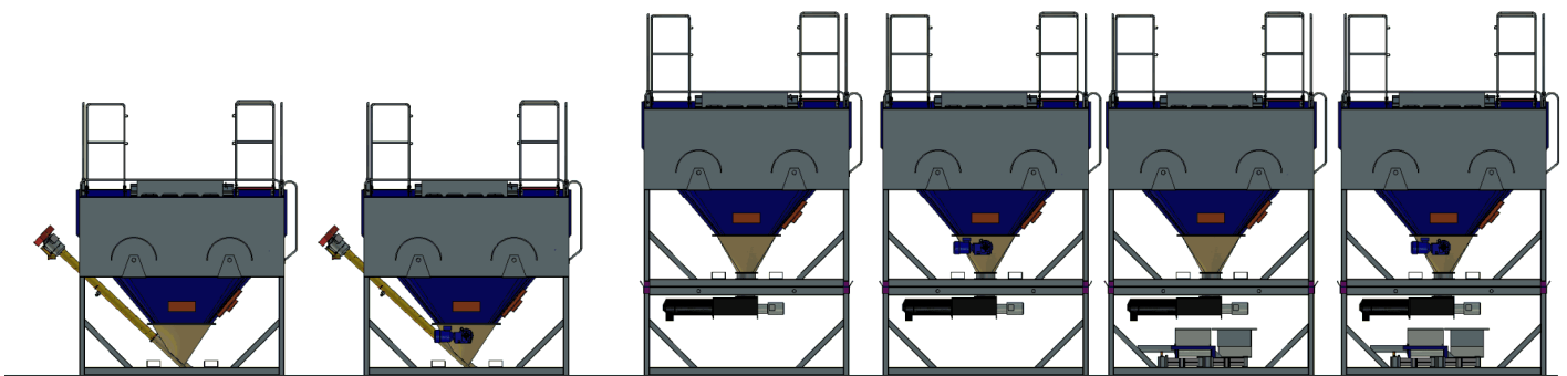
HUVUDMÅTT STORBEHÅLLARE SP10
